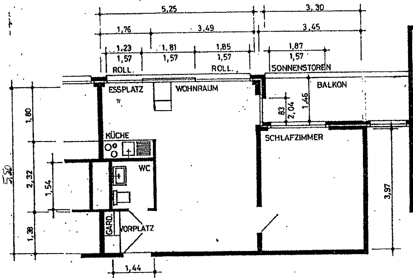
GRUNDRISS 2 - ZIMMERWOHNUNG
